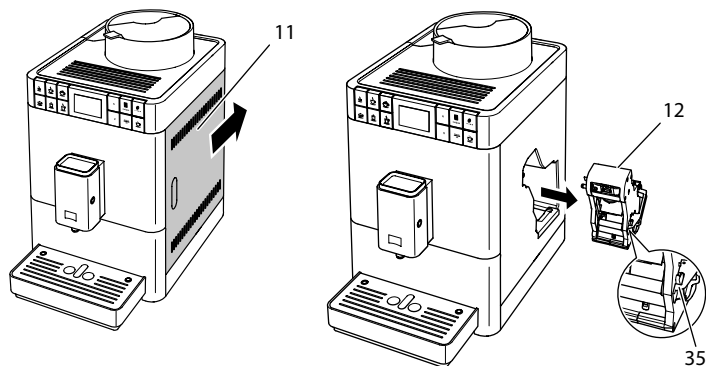
Abb. 17: Brühgruppe entnehmen
